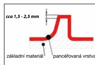
pancéřování celého povrchu šneku
